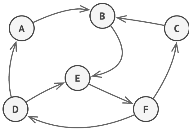
Конечный автомат.
